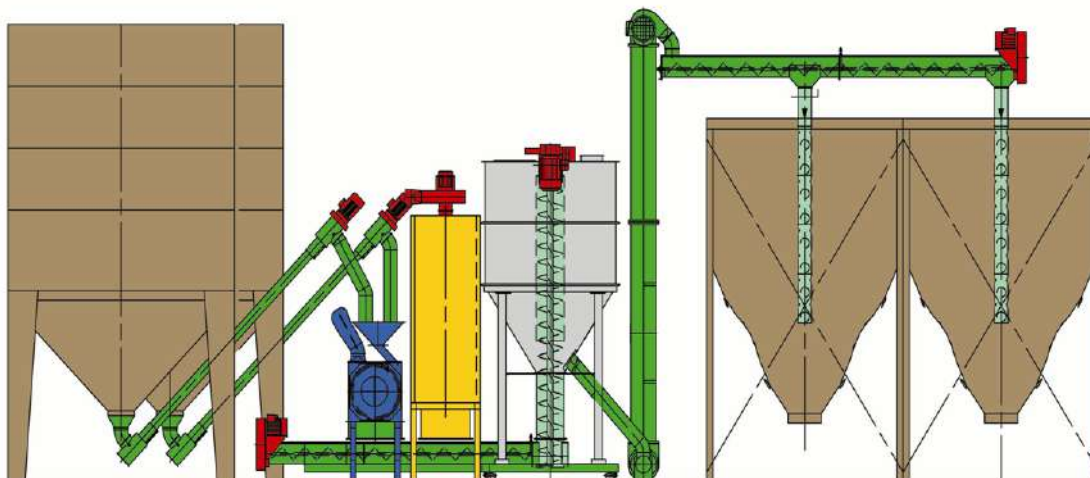
Установка WIDOMIX с мельницей BHOS (без воздухоудвки)
